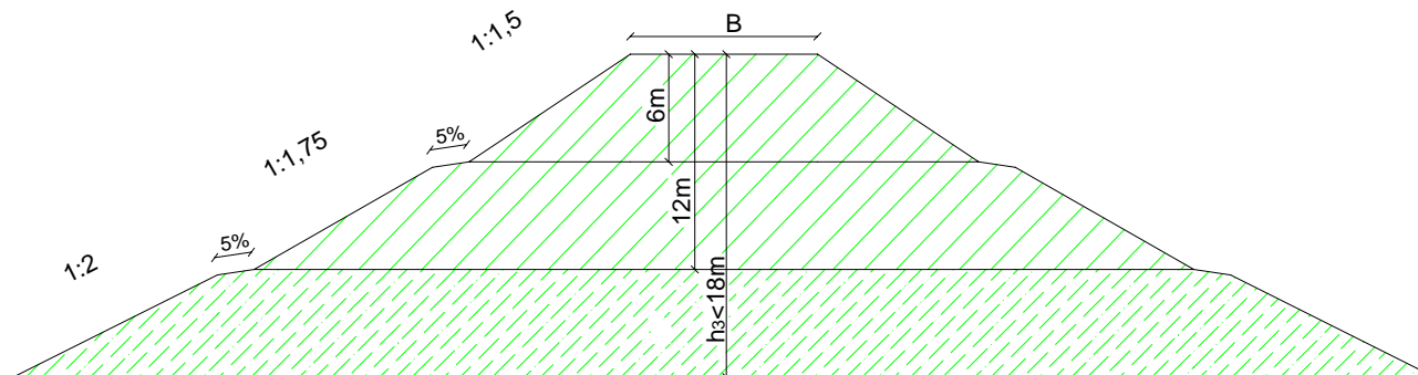
Nasyp do 18 m
