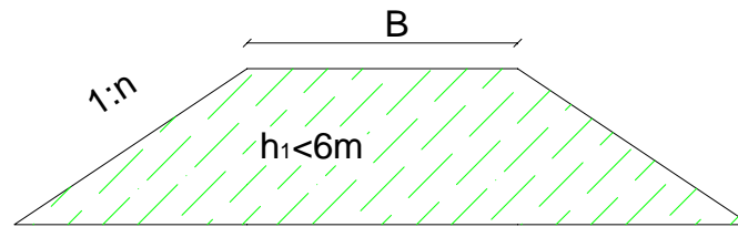
Nasyp do 6 m
