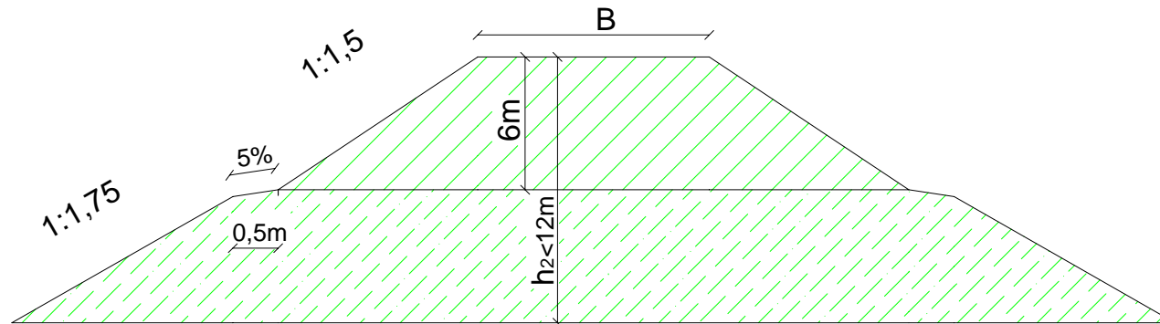
Nasyp do 18 m
